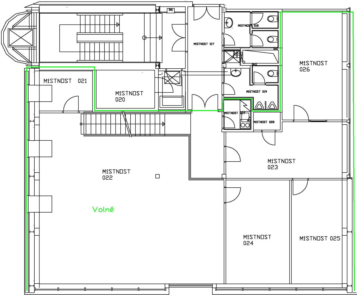
V. patro levá budova (nástavba) 255m2 + 39m2
